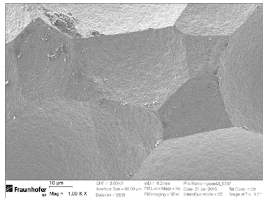
Mit chemischer Politur, ohne Mikrorisse
