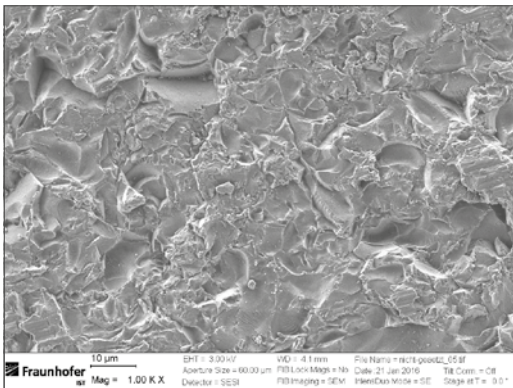
Ohne chemische Politur, Mikrorisse vorhanden
