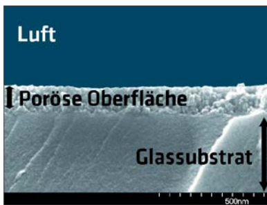
Abbildung: Morphologie der BG-TE Oberfläche auf einem 4,0 mm Glassubstrat Quelle: Fraunhofer ISE
